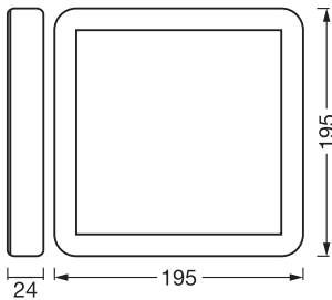
ORBIS QUICKFIX195X19516WCLICKD830
