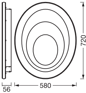
ORBIS SPIRAL OV 720 59W830 CLDIM GR
