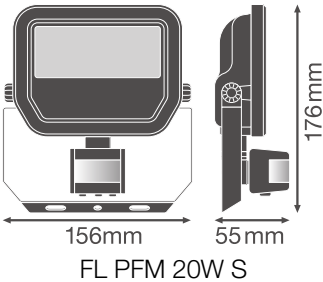
FL PFM 20W S
