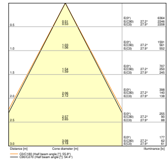
UB WL VARIO RD 29W ML 822 BK 55D Down
