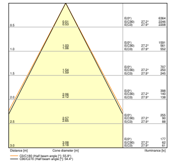
UB WL VARIO RD 29W ML 822 GY 55D Down
