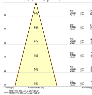
UB WL VARIO RD 29W ML 827 GY 30D Down
