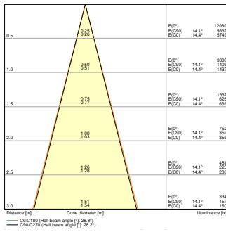
UB WL VARIO RD 29W ML 822 GY 30D Down
