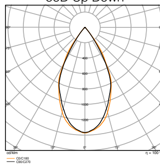
UB WL VARIO RD 29W ML 822 GY 55D Down
