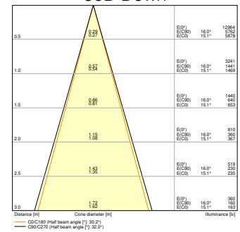
UB WL VARIO RD 29W ML 827 GY 55D Down
