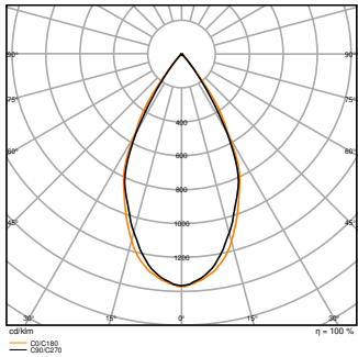
UB WL VARIO RD 29W ML 827 GY 55D Down
