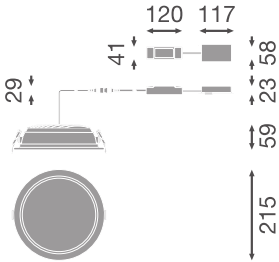
DL CMFT HE D200 P 25W ML
