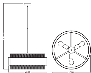
DECOR HORNET PENDANT 3XE27
