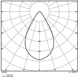
HB DA P 75W 840 70DEG IP66
