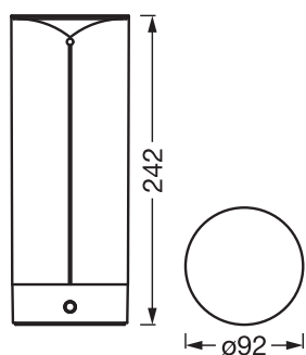
ENDURA STYLE DEC FIL TABLE USB IP54
