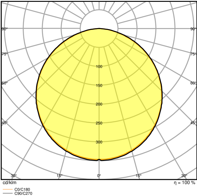
PL CMFT 600 P 28W 830 PS
