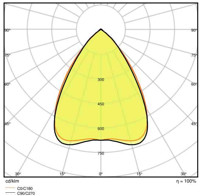
LN INDV D 1500 25W 4000K
