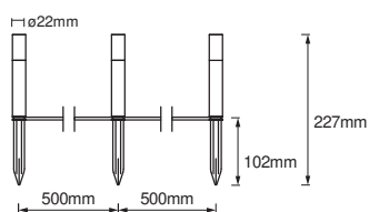
SMART WIFI GARDPOLE MINI RGBW 3PEXT
