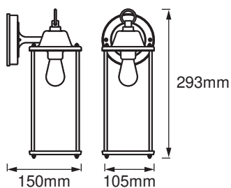
ENDURA CLASSIC LANTERN SQ M E27 BK
