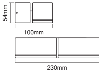
PG ENDURA STYLE Mini Spot II MiPRC
