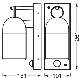
ENDURA CLA COWBELL W S E27 IP65 DG
