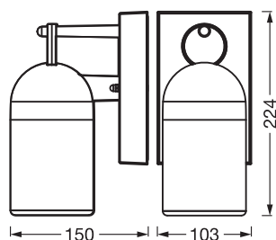
ENDURA CLA COWBELL W E27 IP65 DG
