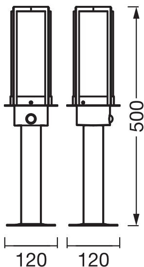
ENDURA CLA HAGEN 50 S E27 IP44 DG
