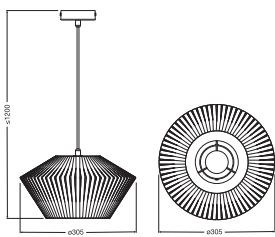
DECOR STRIPES PENDANT 305 1XE27 BG
