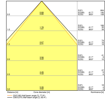
PL CMFT 600 P 33W 840 U19 DALIVR EM CONVERSION BOX
