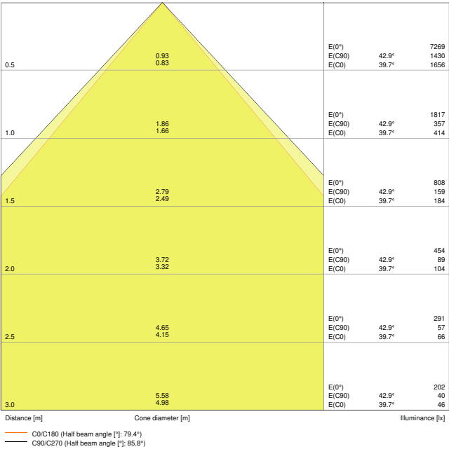
PL PFM 625 30W 3000K UGR19 LDT
