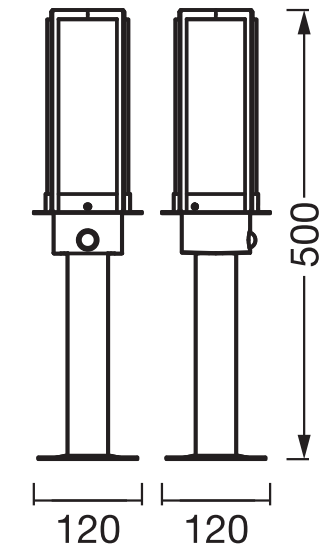
ENDURA CLA HAGEN 50 S E27 IP44 DG
