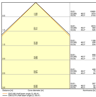
LN INV DI 1500 P 69W 940 DA EL WT 1400mA
