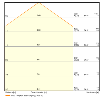
BLKH 250 P 6.5W 830 820lm
