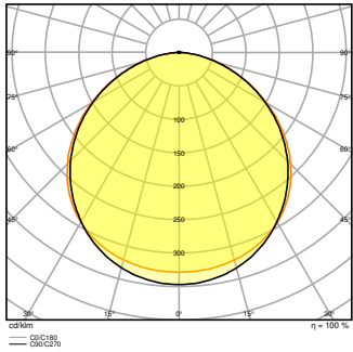
PL CMFT 1200 P 33W 840 DALIVR
