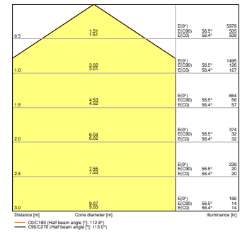
PL CMFT 600 P 33W 865 DALIVR
