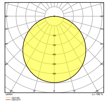
PL CMFT 600 P 33W 830 DALIVR
