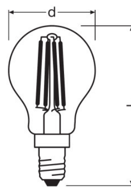
P CLAS P 40 4.5 W/2700K E14
