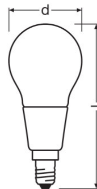
P CLAS P 40 FR 5 W/2700K E14, P CLAS P 60 FR 6.5 W/2700K E14
