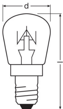
SPC.T CL 25 W 230 V E14
