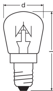
SPC.T FR 10 W 225 V E14, SPC.T CL 15 W 230 V E14, SPC.T CL 25 W 230 V E14
