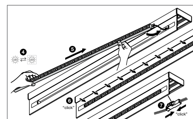
Vervanging van de lichtbron
