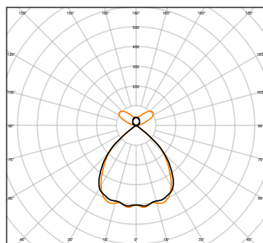
LN INV 1500 D/I 69W/930 PS
