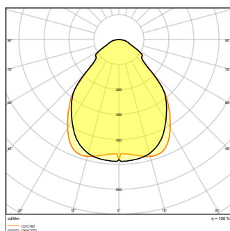
PL CMFT 1200 33W/840 UGR19 PS Lichtstroomselectie met Multi Lumen switch (CRI80 versies)
