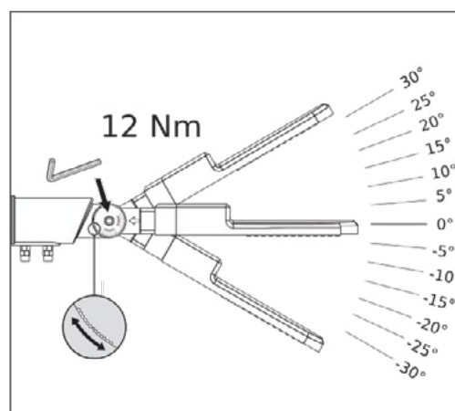
Kantelverstelling
