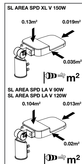
Invloed wind
