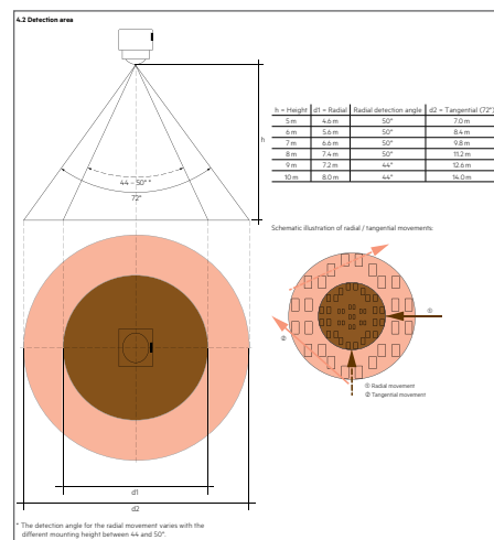
Detectiebereik
