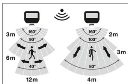
Sensor-detectiezones
