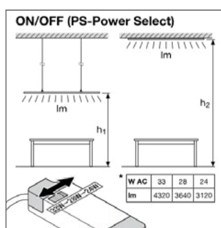
PL CMFT 1200 33W/840 UGR19 PS Lichtstroomselectie met Multi Lumen switch (CRI80 versies)
