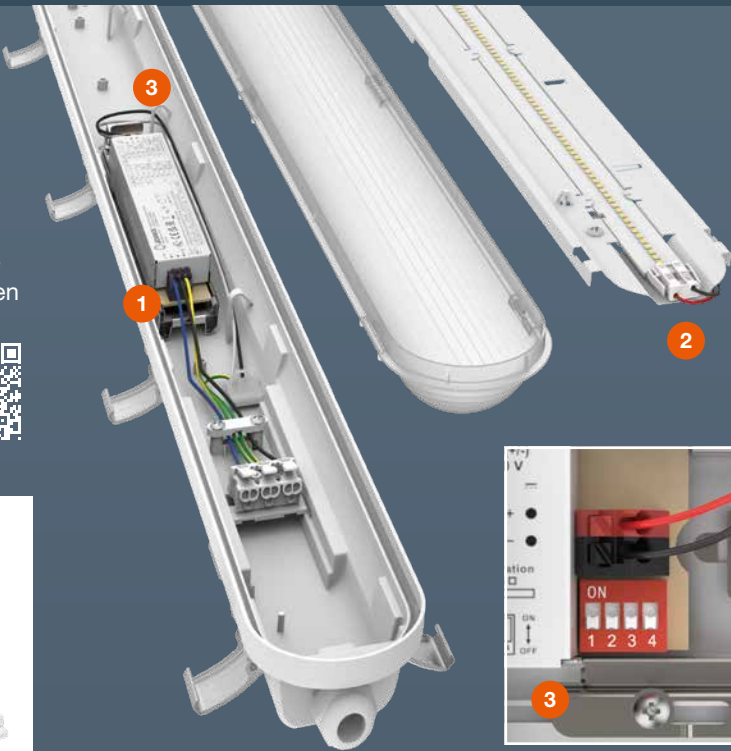
DIP switch voor het instellen van de vermogensstappen
