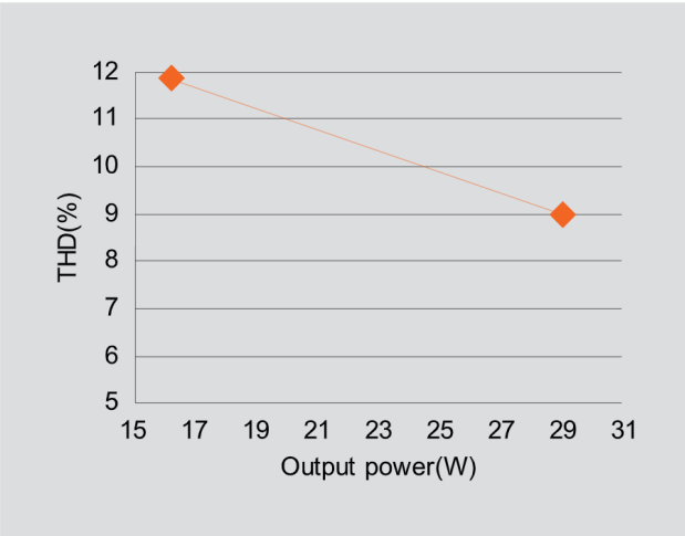
28W THD
