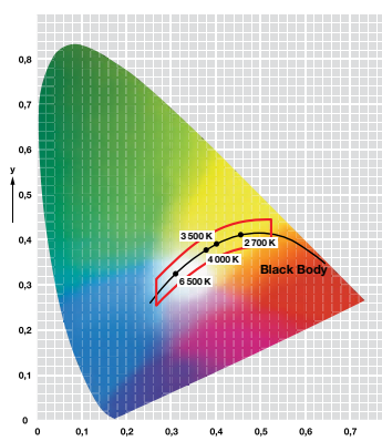
Triangolo dei colori: intervallo di bianco definito dello spettro dei colori delle sorgenti luminose in conformità alle normative UE
