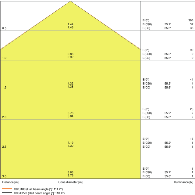
SF BLKH 250 10W3000K S BK IP65 EM discharge LDT
